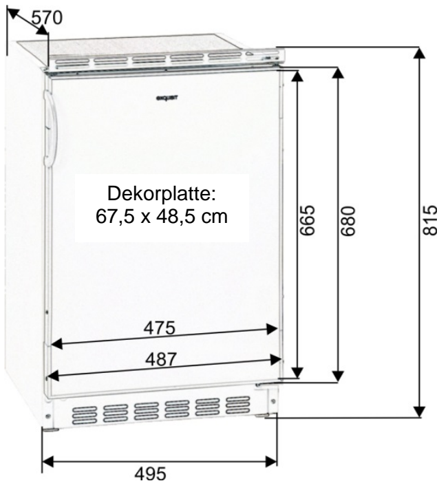
Unterbau-skizze
